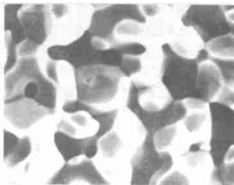
图1 钨骨架断口 SEM 照片 3 600 ×
