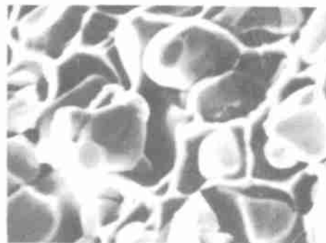
图2 钨铜(10)断口 SEM 照片 3 600 ×
